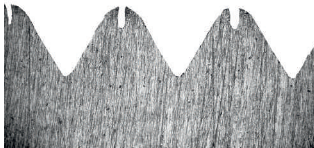
Gwint wygniatany
