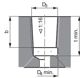
Otwór wstępny zalecany przy otworach nieprzelotowych
